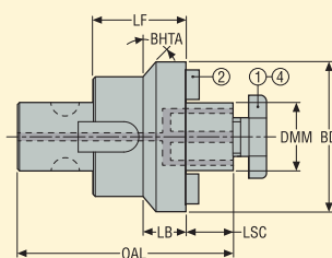
Конструкция 2
