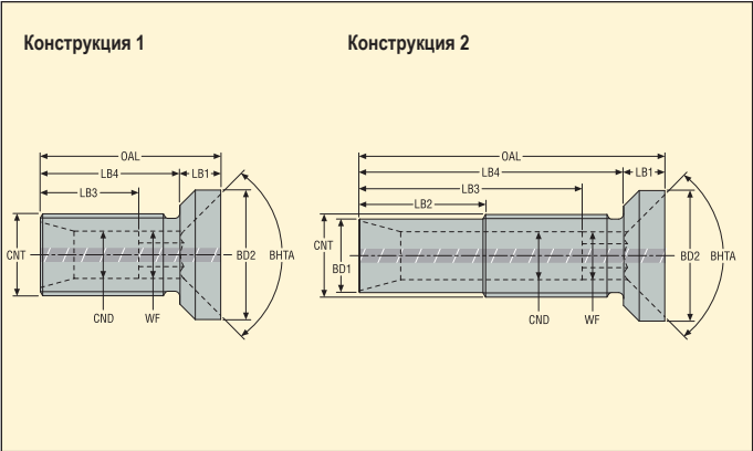
• MQL с коническим соединением, соответствует DIN 69090-3
