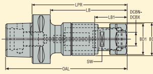
Конструкция 1
