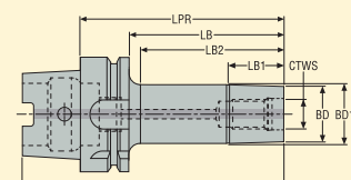
Конструкция 2 (5821)
