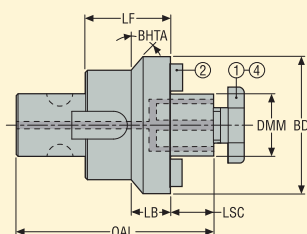
Конструкция 2
