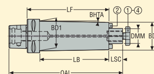
Конструкция 2 (5556)
