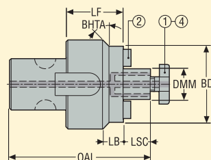
Конструкция 1
