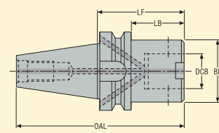
Конструкция 2
