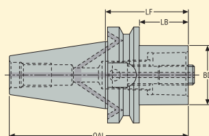
Конструкция 2
