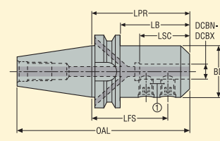
Конструкция 2
