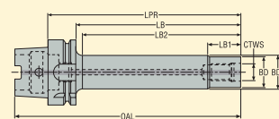
Конструкция 2 (К821)
