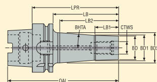
Конструкция 1 (5820)
