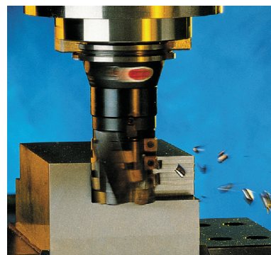
Силовое фрезерование с модульной системой Graflex®: удельный сьем металла 432 см³/мин
