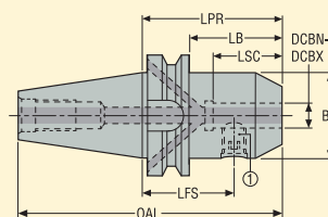
Конструкция 1
