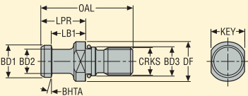
Конструкция 2
