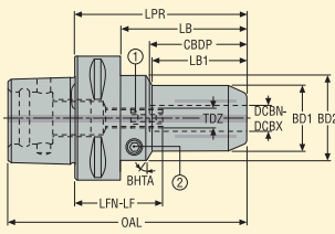
Конструкция 2
