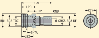
Конструкция 2
