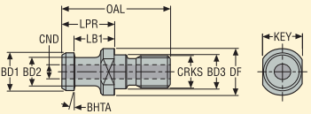
Конструкция 2
